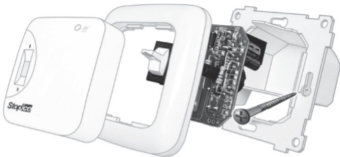
Рис. 4. Сборка повторителя-реле
