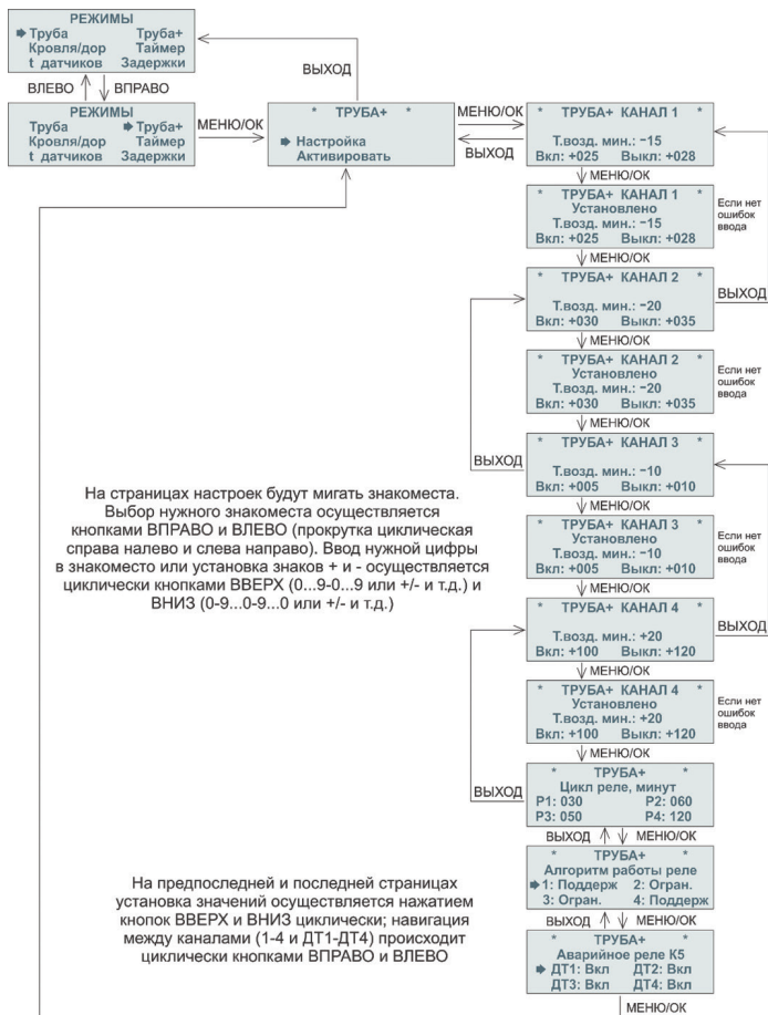
Рисунок 13. Настройка режима «Труба+»
