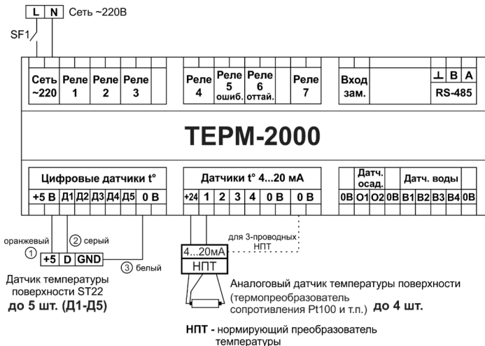
Рисунок 23. Схема подключения ТЕРМ-2000 в режиме «t датчиков»
