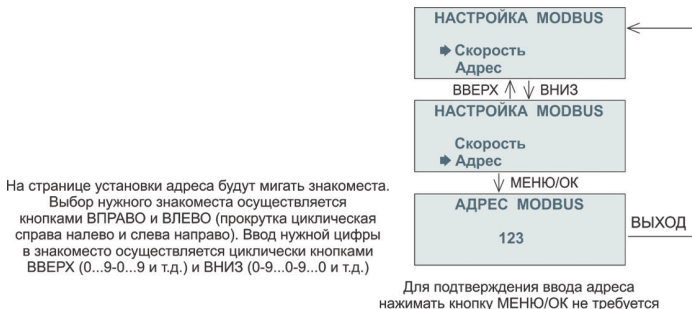
Рисунок 28. Установка адреса устройства в сети MODBUS
