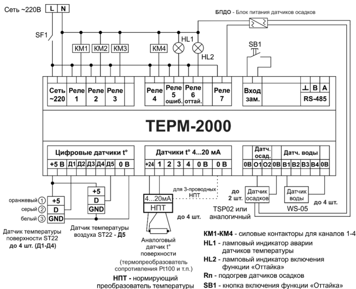
Рисунок 15. Схема подключения ТЕРМ-2000 в режиме «Кровля/дор»
