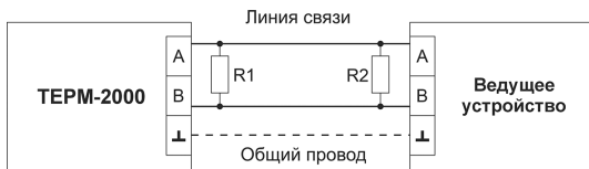
Рисунок 29. Схема соединения ТЕРМ-2000 с ведущим устройством по интерфейсу RS-485 для уменьшения влияния электромагнитных помех
