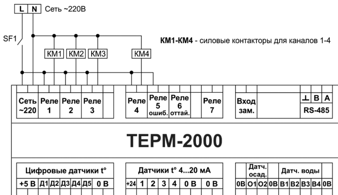
Рисунок 19. Схема подключения ТЕРМ-2000 в режиме «Таймер»
