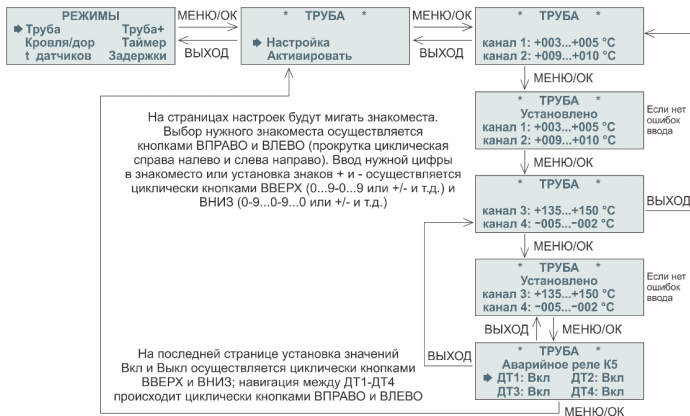
Рисунок 9. Настройка режима «Труба»
