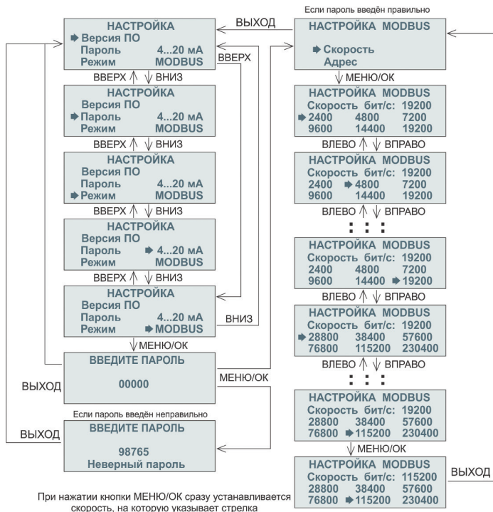
Рисунок 27. Смена предустановленной скорости MODBUS с 19200 кбит/с на 115200 кбит/с
