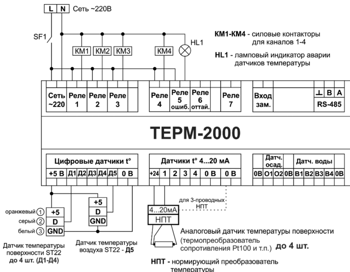
Рисунок 11. Схема подключения ТЕРМ-2000 в режиме «Труба+»
