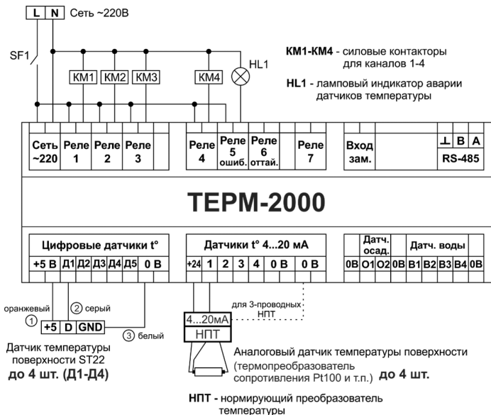
Рисунок 8. Схема подключения ТЕРМ-2000 в режиме «Труба»
